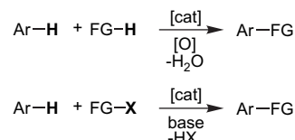
Scheme 2. Aromatic C–H functionalisation.
