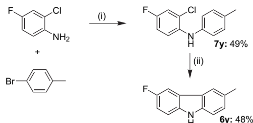
Scheme 11. Conditions: (i) 5 (1 mmol), ArBr (1 mmol), NaO t Bu (5 mmol), Pd(OAc) 2 (5 mol %), [HP t Bu 3 ][BF 4 ] (7 mol %), toluene, Δ, 18 h. (ii) 7 (0.5 mmol), Pd(OAc) 2 (5 mol %), [HP t Bu 3 ][BF 4 ] (7 mol %), NaO t Bu (2.5 mmol), 1,4-dioxane, Δ, 18 h.
