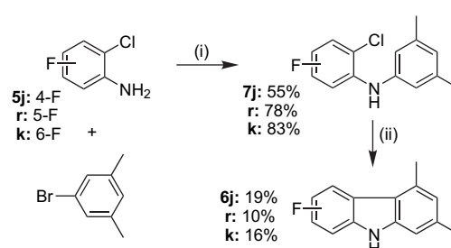
Scheme 10. Conditions: (i) 5 (1 mmol), ArBr (1 mmol), NaO t Bu (5 mmol), Pd(OAc) 2 (5 mol %), [HP t Bu 3 ][BF 4 ] (7 mol %), toluene, Δ, 18 h. (ii) 7 (0.5 mmol), Pd(OAc) 2 (5 mol %), [HP t Bu 3 ][BF 4 ] (7 mol %), NaO t Bu (2.5 mmol), 1,4-dioxane, Δ, 18 h.
