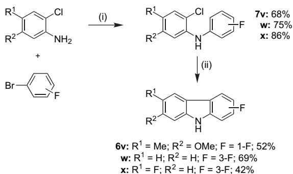
Scheme 9. Conditions: (i) 5 (1 mmol), ArBr (1 mmol), NaO t Bu (5 mmol), Pd(OAc) 2 (5 mol %), [HP t Bu 3 ][BF 4 ] (7 mol %), toluene, Δ, 18 h. (ii) 7 (0.5 mmol), Pd(OAc) 2 (5 mol %), [HP t Bu 3 ][BF 4 ] (7 mol %), NaO t Bu (2.5 mmol), 1,4-dioxane, Δ, 18 h.
